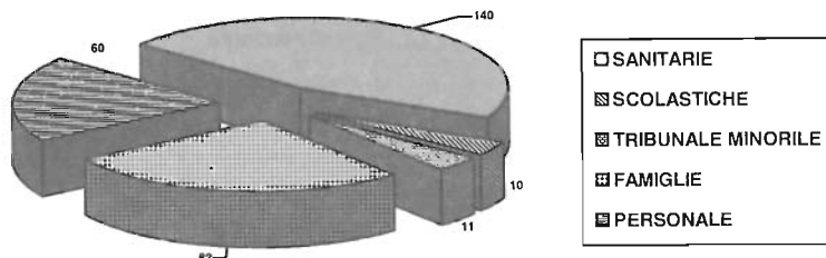
Fig. 3. Strutture invianti
